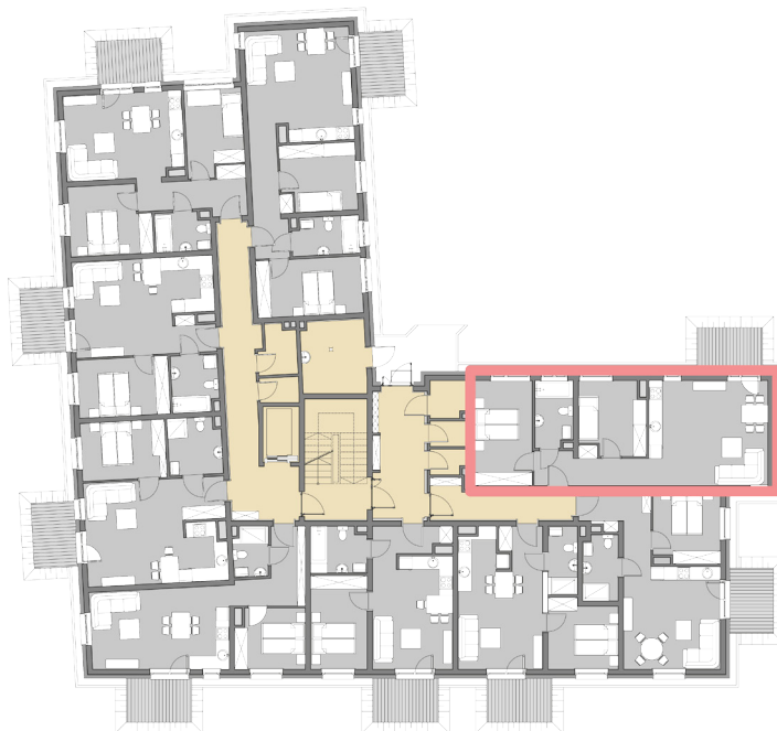
RZUT KONDYGNACJI: PARTER
